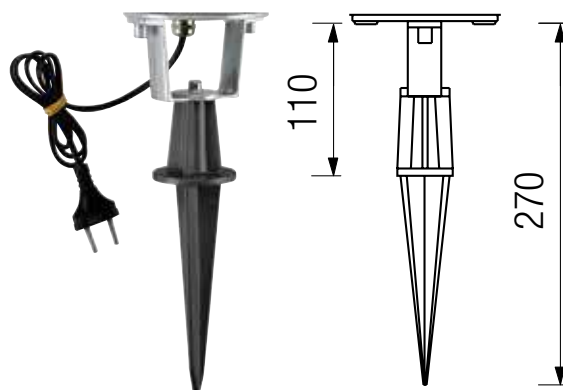
Installazione a terra con picchetto Ground fixing with spike
